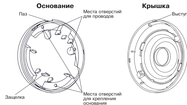
Рисунок 2 – Основание и крышка извещателя
