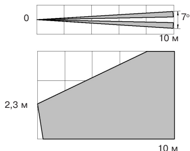
Рисунок 1 – Диаграмма зоны обнаружения
