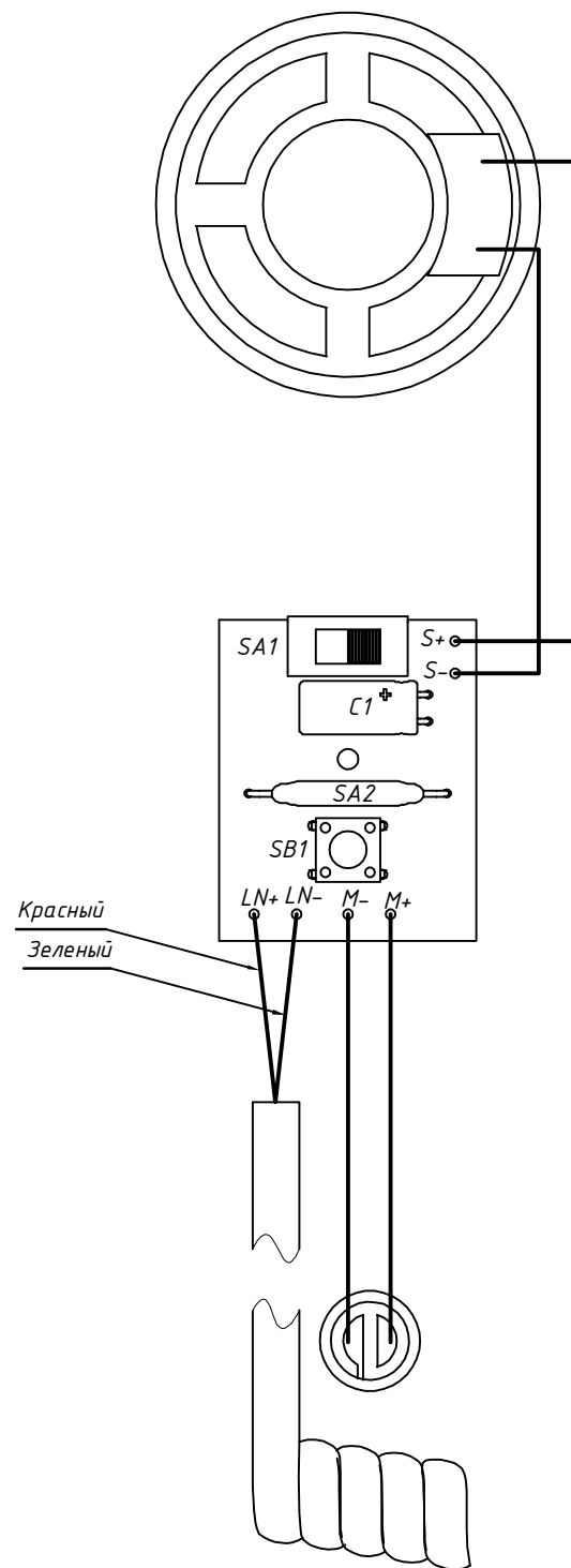
Плата УКП-7(М) Сборочный чертеж
